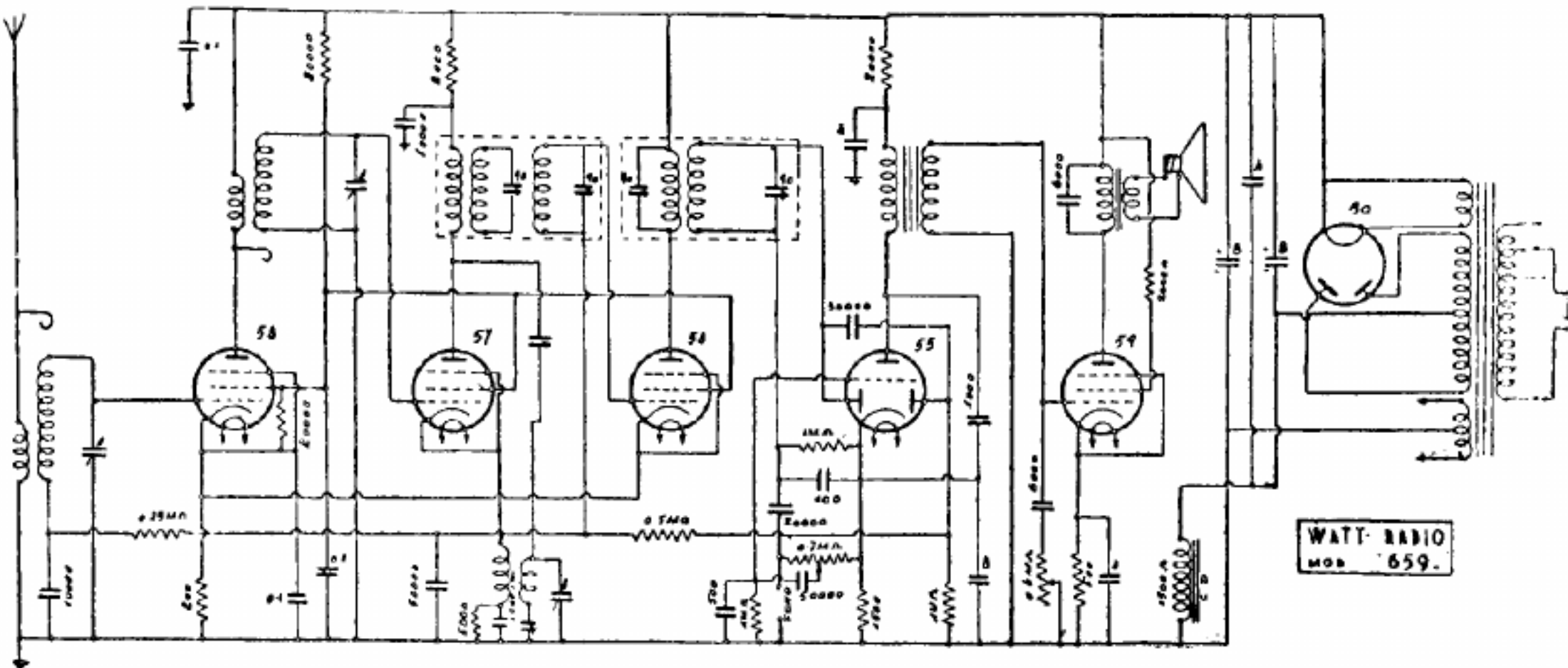
WATT RADIO. — Modello « 659 » , Produzione 1934. • Media frequenza: 175 kc.
